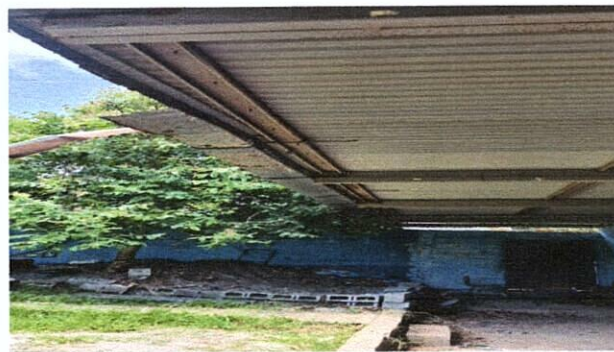
Foto 4: SUSTITUCION DE TECHO DE LAMINA TROQUELADA CAL. 26
