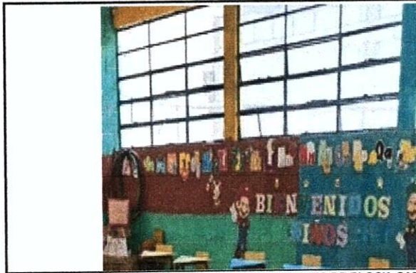
FOTO 1: SUSTITUCION DE VENTANA CON CERRAMIENTO DE BLOCK, SABIETA Y REPELLO, MEJORAMIENTO EN PARED Y TALLADO PARA VENTANA, SUSTITUCION DE VENTANA POR VENTANA DE PVC BLANCO, SUSTITUCION E INSTALACIÓN DE BALCÓN DE ESTRUCTURA METÁLICA
