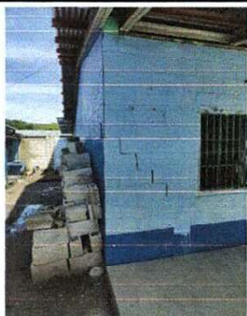
Foto 1: Mejoramiento y Reforzamiento de muro en módulo
