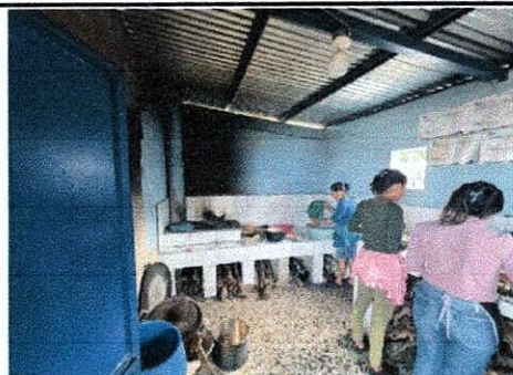
Foto 5: MEJORAMIENTO DE ESTUFA RURAL Y MUEBLE DE COCINA CON INSTALACIÓN DE AZULEJO EN ÁREA DE COCINA
