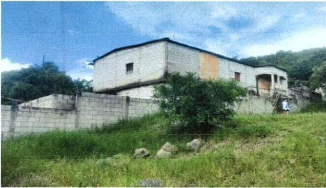
Foto 1: Mejoramiento de muro perimetral de block con tubo hg y malla galvanizada a 1.5 metros
