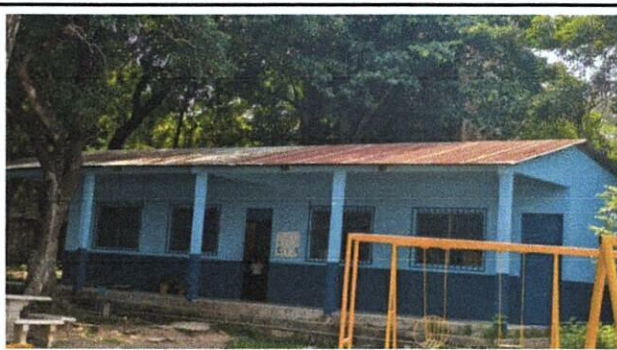
Foto 2: SUSTITUCIÓN DE TECHO DE LÁMINA ACANALADA CON ESTRUCTURA METÁLICA POR LÁMINA TROQUELADA DE ALUZINC CALIBRE 26, MANTENIMIENTO A ESTRUCTURA E INSTALACIÓN DE CAPOTE.
