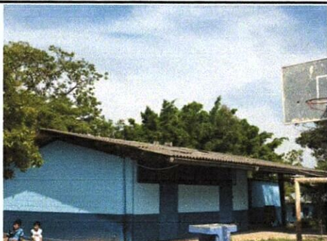
Foto 1: SUSTITUCIÓN DE TECHO DE DURALITA CON ESTRUCTURA METÁLICA POR LÁMINA TROQUELADA DE ALUZINC CALIBRE 26
