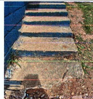
Foto 6: Reparación de gradas de concreto
