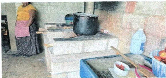
Foto 3: Sustitución de estufa rural (completa) incluye chimenea y plancha de metal
