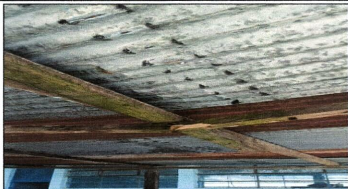
Foto1: SUSTITUCIÓN DE ESTRUCTURA DE SOPORTE DE MADERA POR METAL, MEJORAMIENTO DE CANAL PVC
