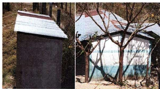
Foto 2: Sustitución de lamina por lamina troquelada aluzinc en modulo de aula, sanitarios y bodega.
