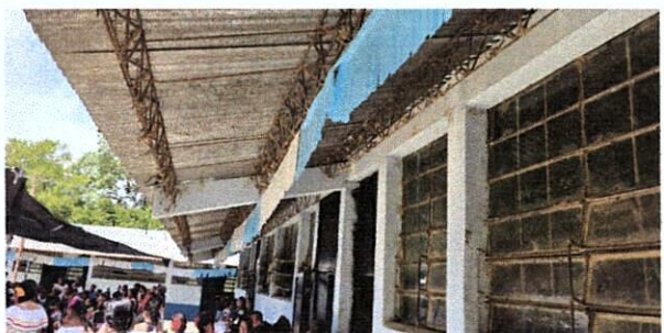
Foto 3: SUSTITUCIÓN DE LÁMINA TROQUELADA CAL. 26
