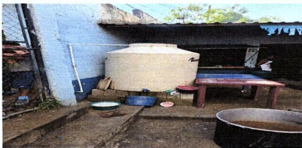
FOTO 5: MEJORAMIENTO DE BASE PARA TINACO
