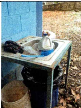
Foto 1: SUSTITUCIÓN CON LAVAMANOS CON PEDESTAL (INCLUYE CONTRALLAVE
