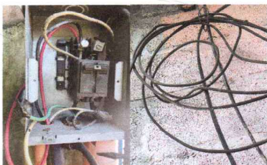
Foto 3: sustitucion de linea principal del sistema electrico
