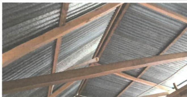
Foto 1: Sustitución de estructura de soporte de madera, por metal
