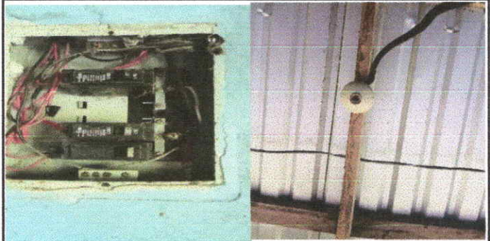
Foto 6: sustitución de plafoneras, tomacorrientes y sustitución de filipones
