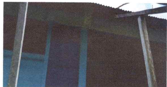
Foto 6: Sustrucción de columnas de madera por columnas de concreto (pasillo exterior del aula)
