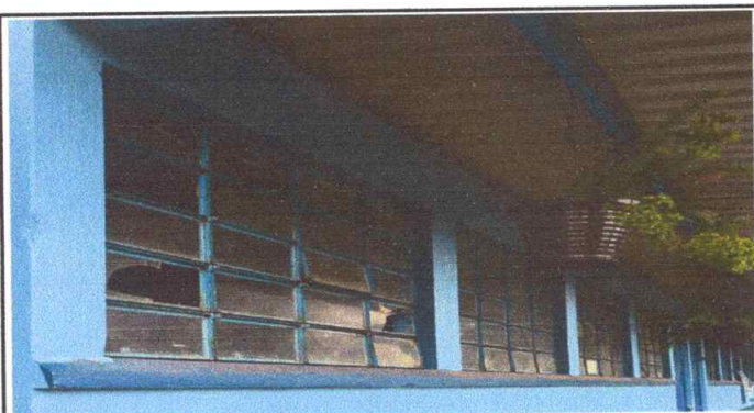
Foto No 3: Sustitución de balcones de metal
