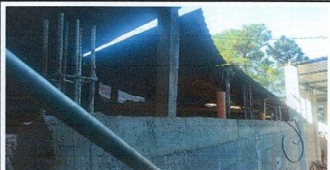
Foto 9.1 Mejoramiento de pared
