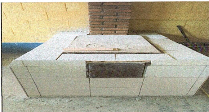
Foto 11: SUSTITUCIÓN DE ESTUFA RURAL (COMPLETA) INCLUYE CHIMENEA Y PLANCHA DE METAL FINALIZADO
