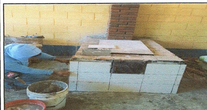
Foto 11: SUSTITUCIÓN DE ESTUFA RURAL (COMPLETA) INCLUYE CHIMENEA Y PLANCHA DE METAL EN PROCESO
