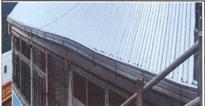
Foto 4: finalización de canal de metal y sustitución de soporte o pescante de metal para canal
