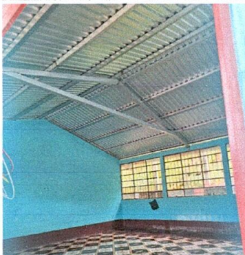
Foto 1: Sustitución de estructura de soporte por metal
