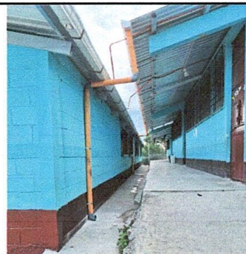
Foto 12: Sustitución de bajada de agua pluvial de metal por tubo PVC 3
