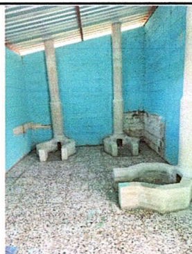
Foto 18: Sustitución de estufa rural completa no convencional
