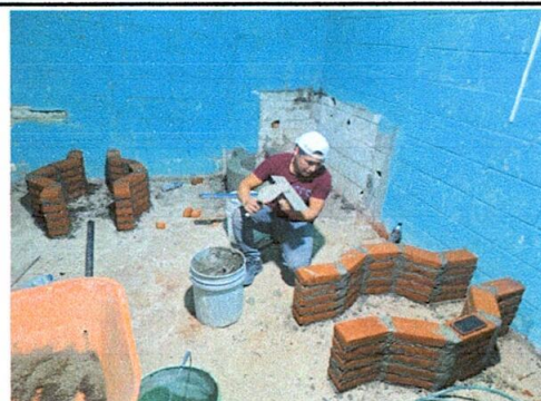
Foto 18: Sustitución de estufa rural completa no convencional
