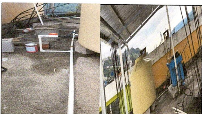
Foto 3: instalación de cisterna y tubería terminada
