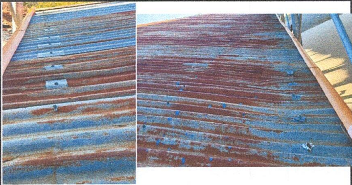
Foto1: CUBIERTA DE LÁMINA: SUSTITUCION DE LAMINA, CAPOTE, ELEMENTOS DE FIJACIÓN
