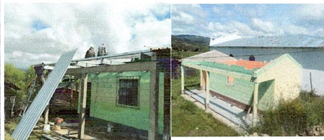
Foto 6: Sustitución de lámina, por lámina troquelada
