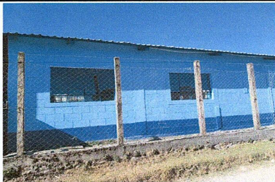
Foto 26: SUSTITUCIÓN DE VENTANAS DE MADERA POR VENTANAS DE METAL Y VIDRIO
