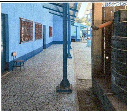
Foto 15: SUSTITUCIÓN DE ESTRUCTURA DE SOPORTE DE MADERA POR METAL
