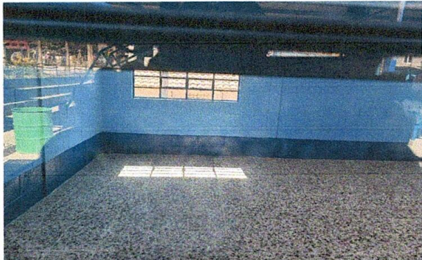
Foto1: SUSTITUCIÓN DE PISO DE TORTA DE CONCRETO POR PISO DE GRANITO
