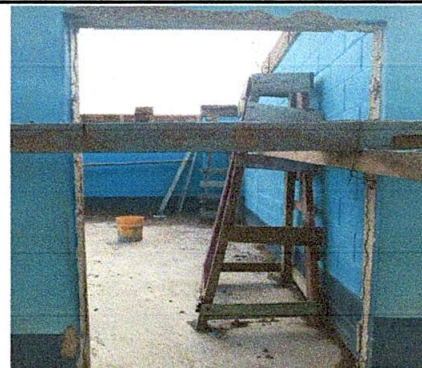
Foto 20: SUSTITUCIÓN DE 3 PUERTAS DE MADERA POR PUERTAS DE METAL
