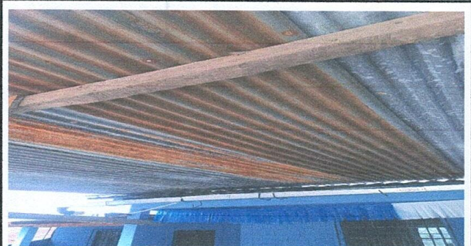
FOTO 3: Sustrución de lámina por lámina troquelada
