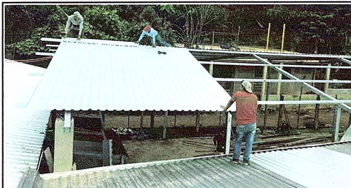
Foto1: Instalación de láminas y capotes
