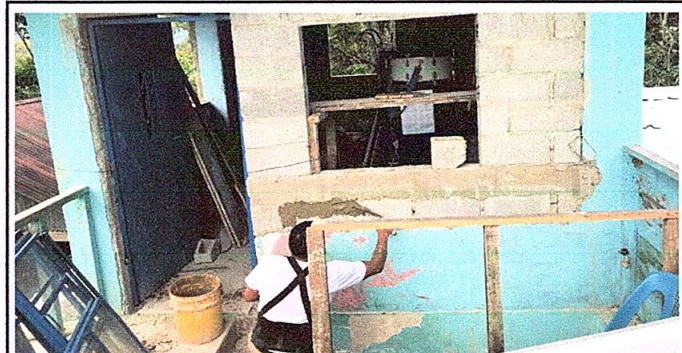
Foto 6: Repello en pared
