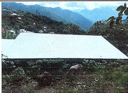
FOTO 1: Sustrucción de lámina, por lámina troquelada aluzinc calibre 26
