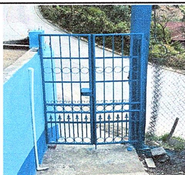
FOTO 5: Sustrucción de portón de metal de 2 mts. de alto x 1.50 mts. de ancho
