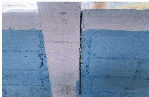
Foto 10: Sellado de grietas y fisuras en muro
