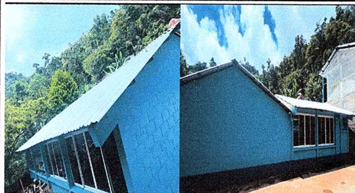
Foto 1: Sustitución de lámina por lámina troquelada aluzinc calibre 26, en cuatro aulas y dirección de la escuela.
