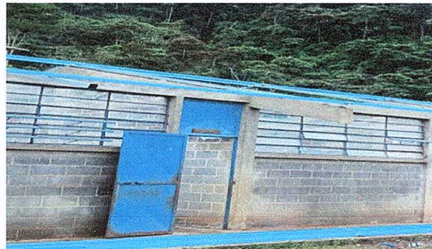
Foto 4: Sustitución de puerta (2.09m de alto * 0.97m de ancho)
