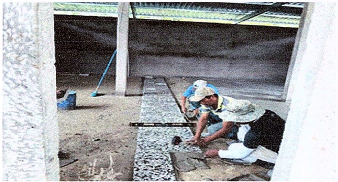
FOTO 3: Sustitución de piso de granito
