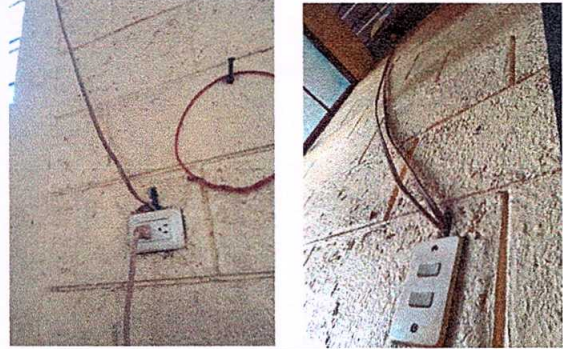
Foto 10: Tomacorrientes e interruptores en mal estado.
