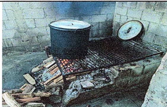
Foto 8: reparacion de cocina. Sustitución de planchas de metal
