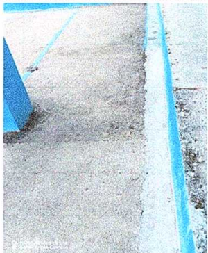
FOTO No. 1: Sustrucción de piso de torta de concreto.
