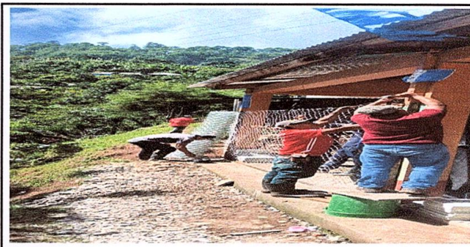
Foto 6: Mejoramiento con tubo HG y malla galvanizada
