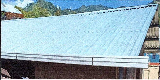
Foto 1: SUSTITUCIÓN DE LÁMINA, POR LÁMINA TROQUELADA ALUZING CALIBRE 26
