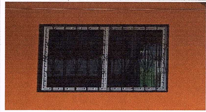
Foto 4: SUSTITUCIÓN DE VENTANAS DE MADERA POR METAL MÁS VIDRIO
