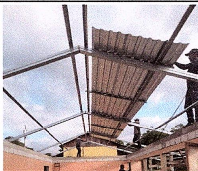
Foto 6: Sustitución de lámina, por lámina troquelada aluzinc calibre 26
