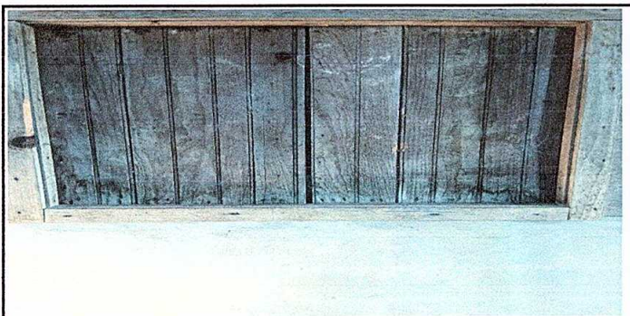
Foto 5: Sustrucción de ventanas de madera por metal mas vidrio (1.10m de alto y 2m de ancho)
