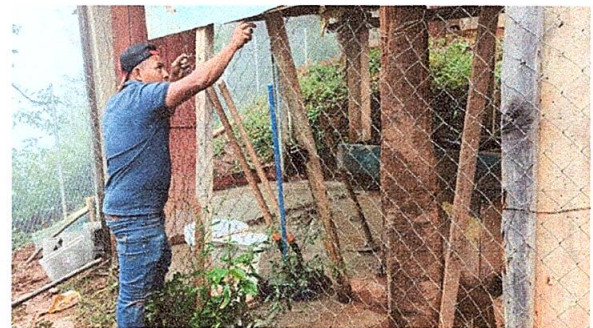
Foto 4: REPARACIÓN DE TUBO HG Y MALLA GALVANIZADA
