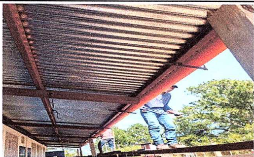
Foto1: INSTALACION SOPORTE DE METAL Y BAJADA DE AGUA PLUVIAL
