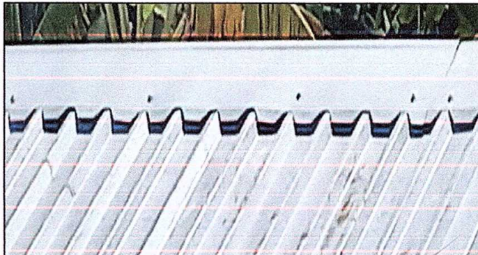
Foto 4: sustitución de capote de lámina para lámina troquelada
