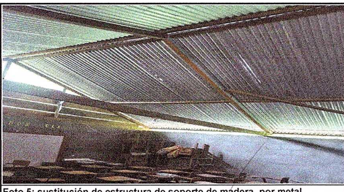
Foto 5: sustitución de estructura de soporte de madera, por metal
