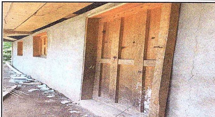
Foto 2: sustitución de puerta (2.10m de alto X 1.00m de ancho)
