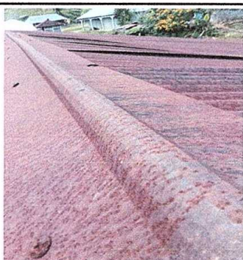
Foto 3: Sustitución de capote de lámina para lámina troquelada
