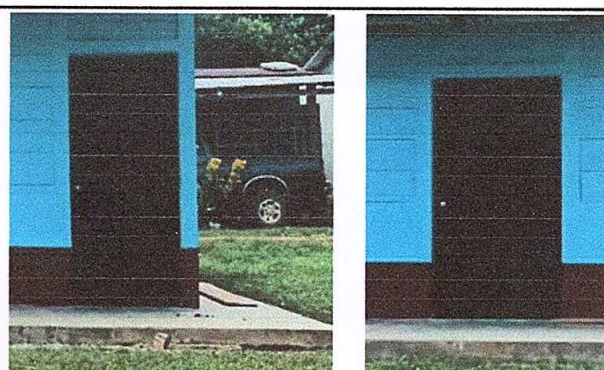
Foto 4: Sustitución de puerta (2m de alto * 1m de ancho)
