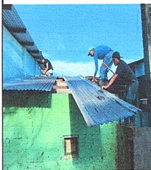
Foto1: Sustitución de lámina, por lámina troquelada aluzinc
