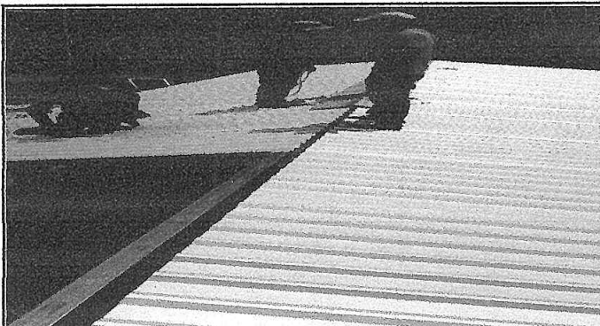
Foto1: sustitución de láminas, por lámina troquelada aluzinc calibre 26
